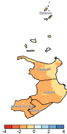
SPEI3 (Nov-Dec-Jan)
