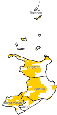
NDVI
